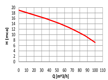
Jelleggörbe 5,5 LE
