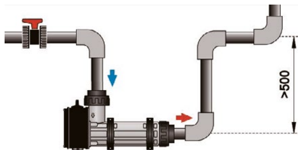
BEÉPÍTÉSI RAJZ
